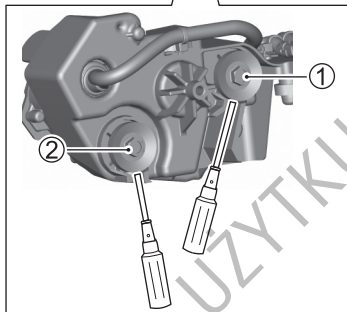
Światło mijania
